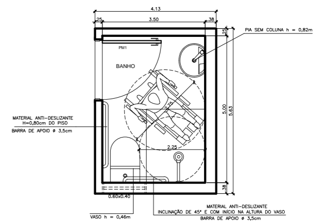
DETALHE 01 BANHO DEF. ESCALA 1:20
